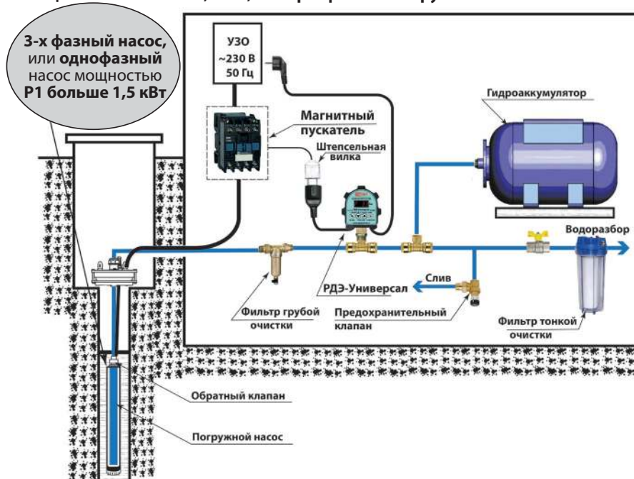
Пример 4. Подключение РДЭ-Универсал для управления однофазным насосом мощностью P1 более 1,5 кВт, или трехфазным погружным насосом.
