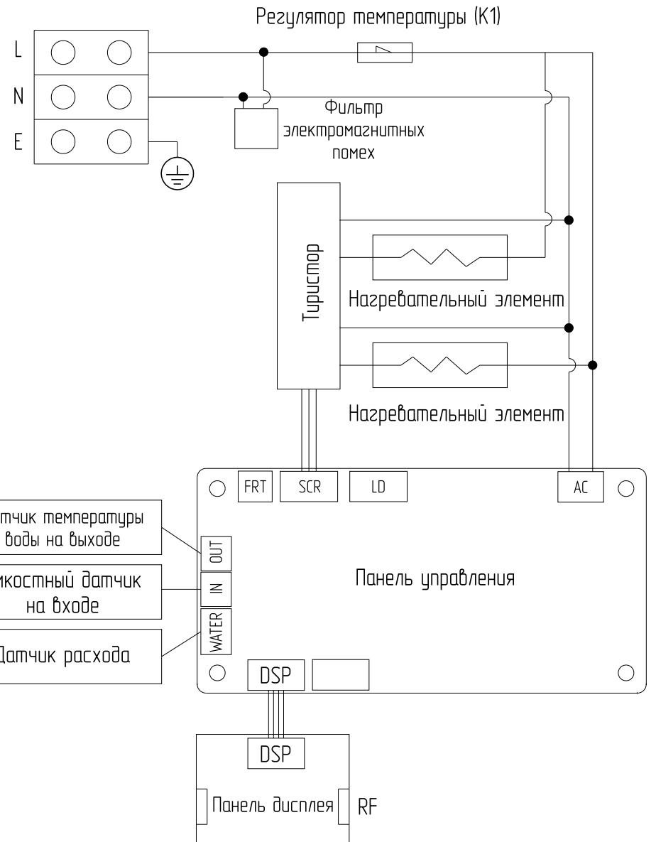
Рис.9 Схема подключения ZOTA JOY 7-9 кВт, 220 В
