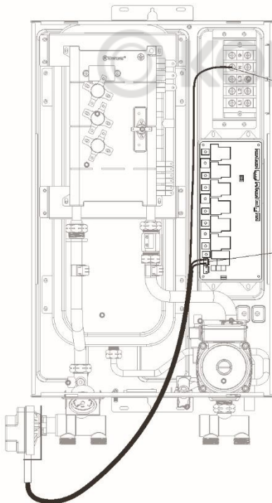
Рис. 17. Подключение трехфазного клапана
