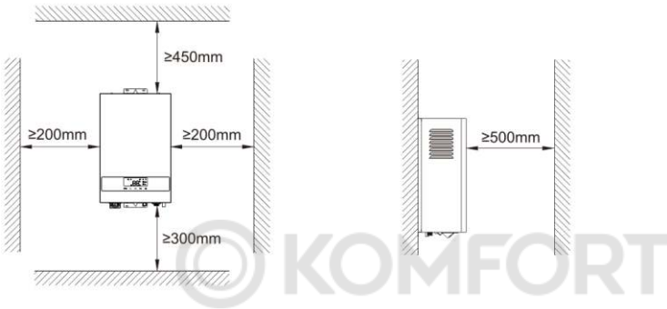
Рис. 4. Минимальные расстояния от электрического котла до поверхностей.
