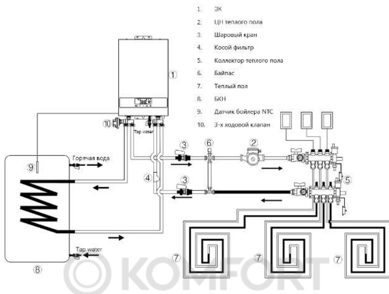
Рис. 20. Схема подключения «ЭК + БКН + Теплый пол».
