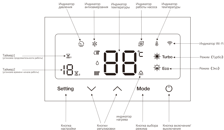
Рис. 3. Панель управления
