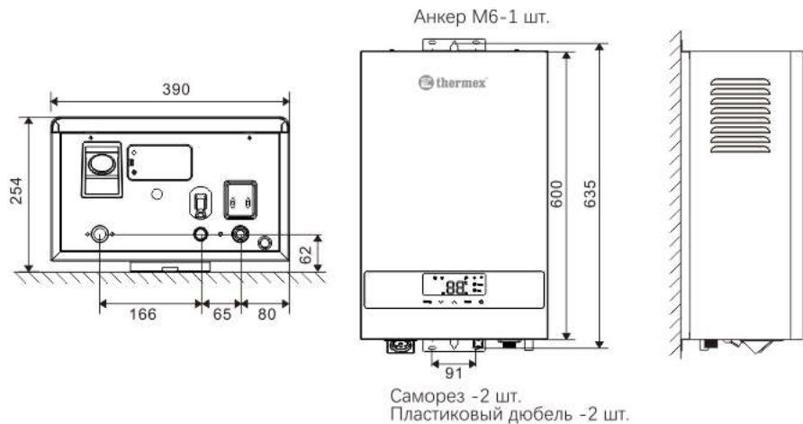
Рис. 5. Монтажные размеры
