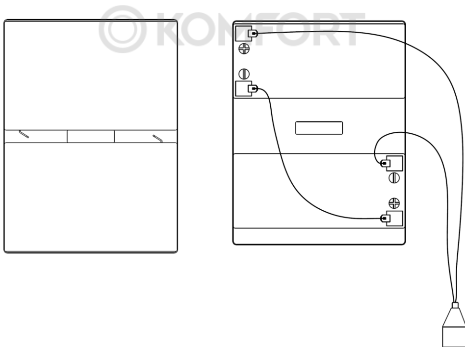
Рисунок 6 — размещение АКБ в лотке
