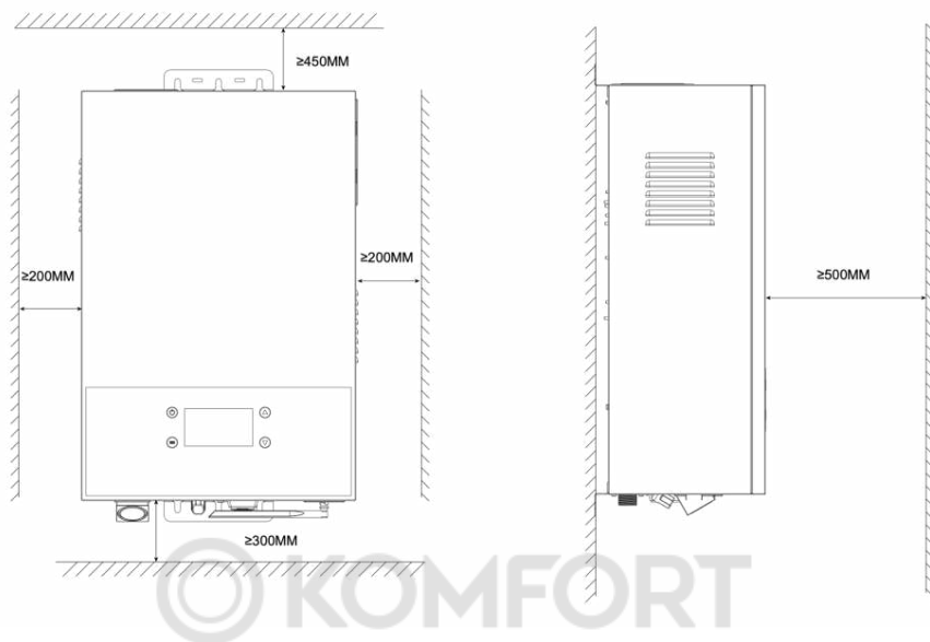
Рис. 4. Минимальные расстояния от электрического котла до поверхностей.
