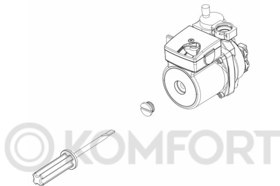
Рис. 20. Проверка насоса
