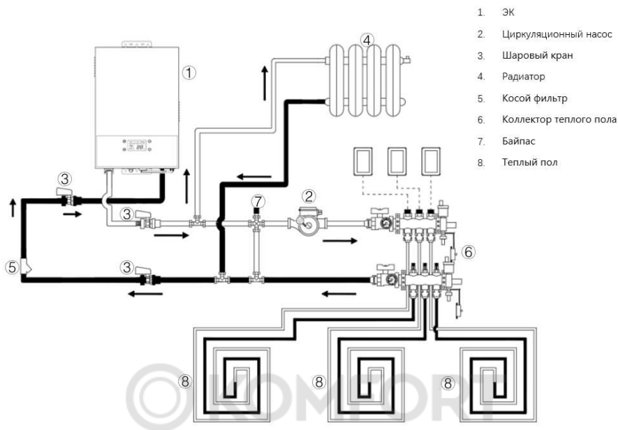
Рис. 7. Схема подключения «радиаторы + теплый пол + ЭК»
