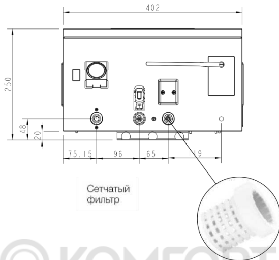
Рис. 19. Сетчатый фильтр
