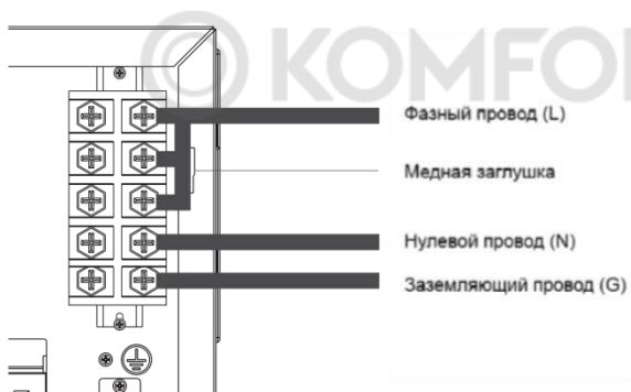
Рис. 10. Однофазное подключение прибора
