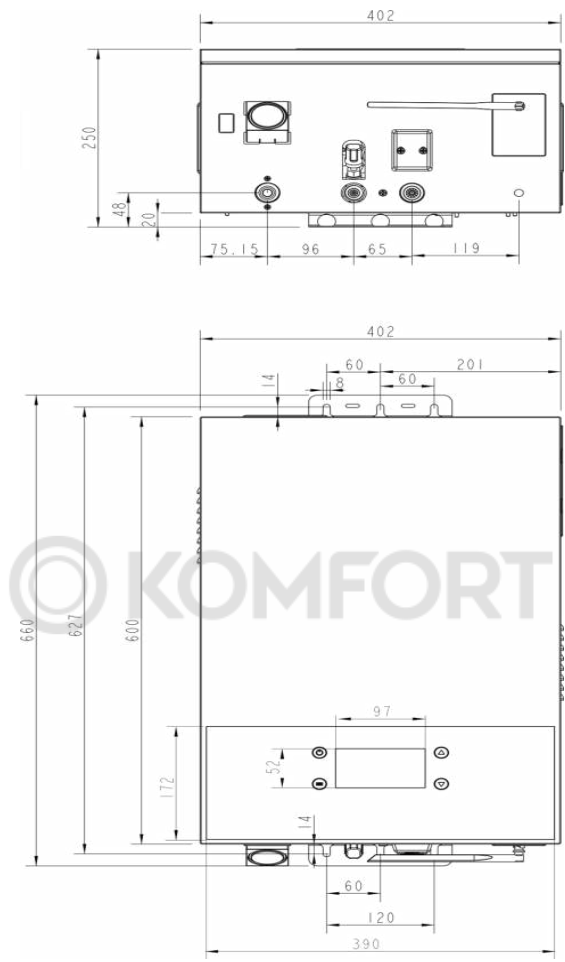
Рис.2. Габаритные размеры
