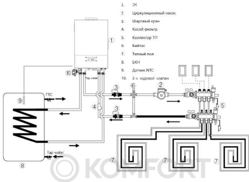
Рис. 16 Схема подключения «ЭЖ + БКН + теплый пол»
