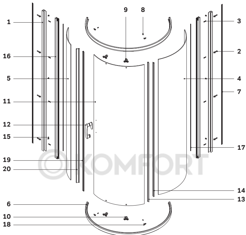
Gehäuse konfiguration / Enclosure configuration / Комплектация ограждения 90x90
