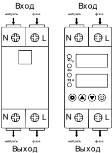
Рис.2 Схема подключения.
