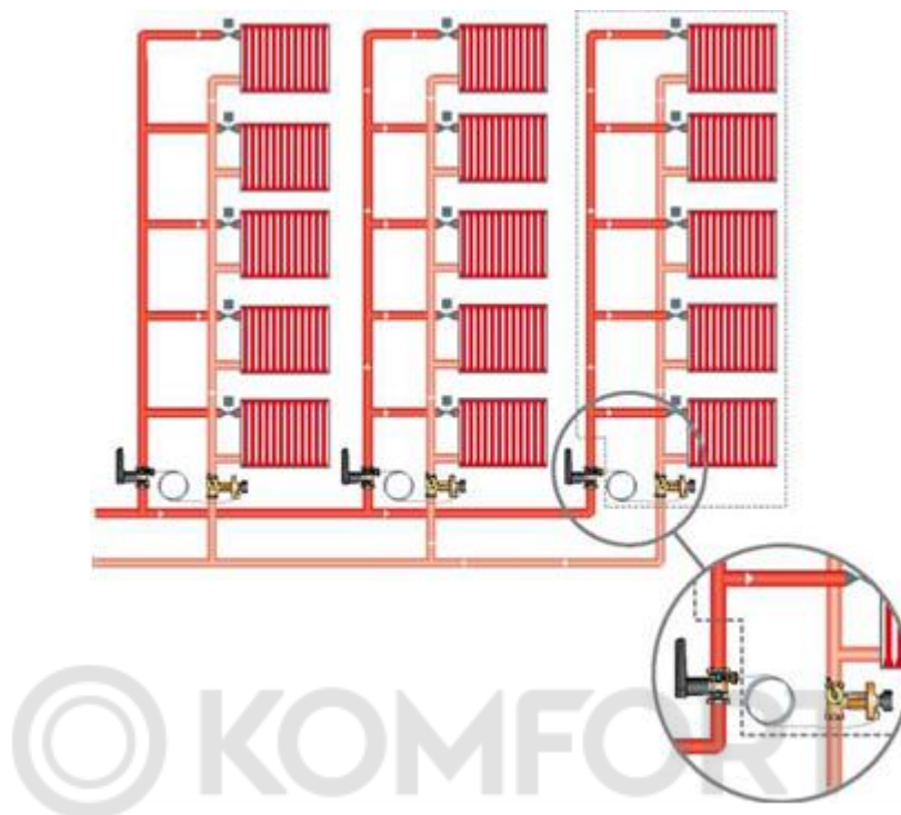
Рис. 2 Двухтрубная стояковая система отопления
