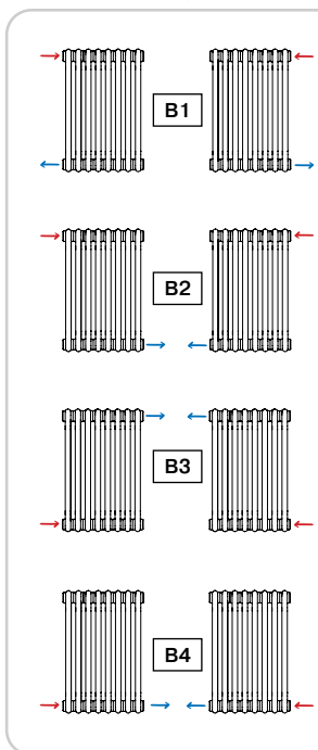
Боковое подключение
