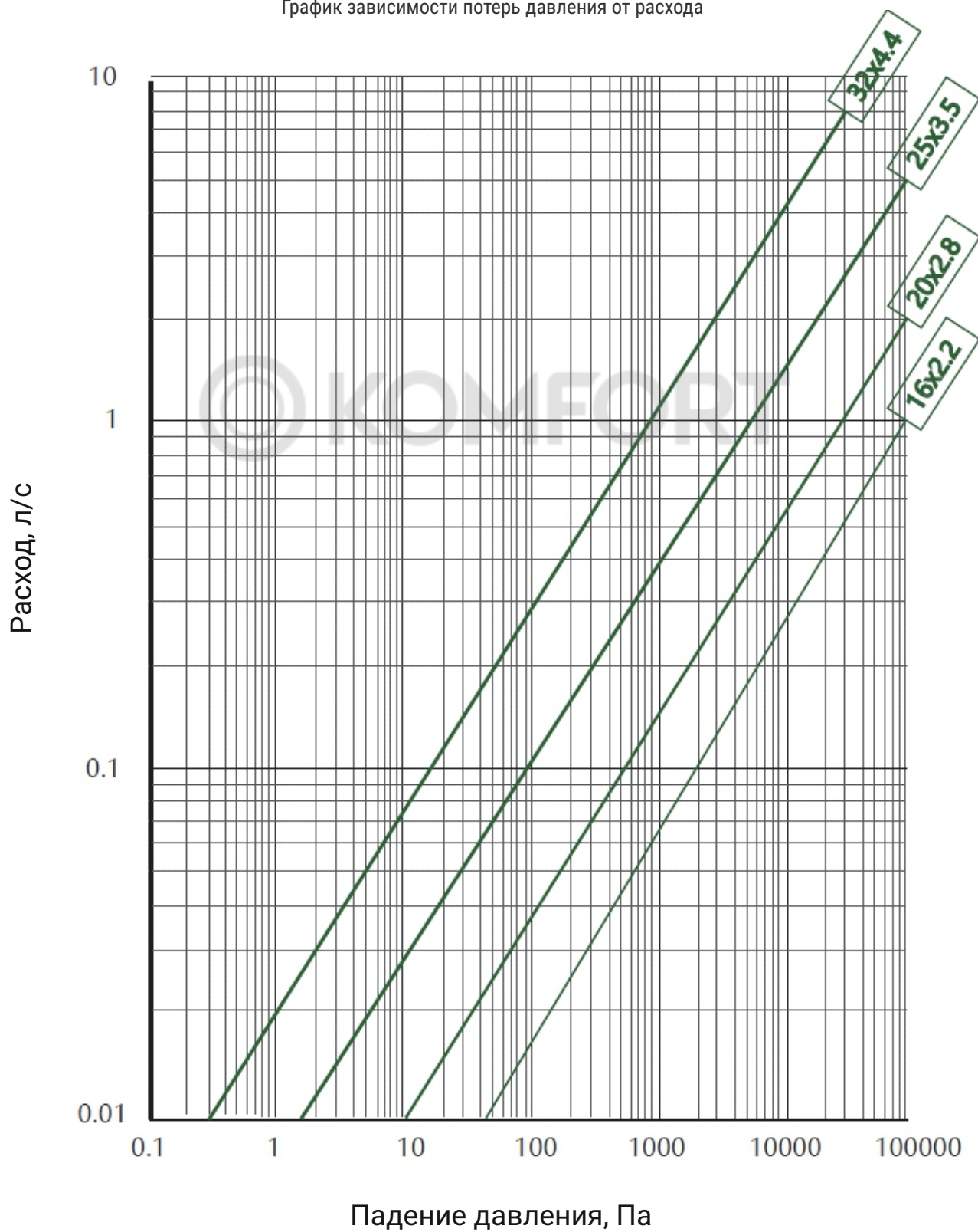
График зависимости потерь давления от расхода
