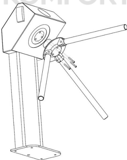
Рисунок 6 установка ступицы со штангами ограничителями.
