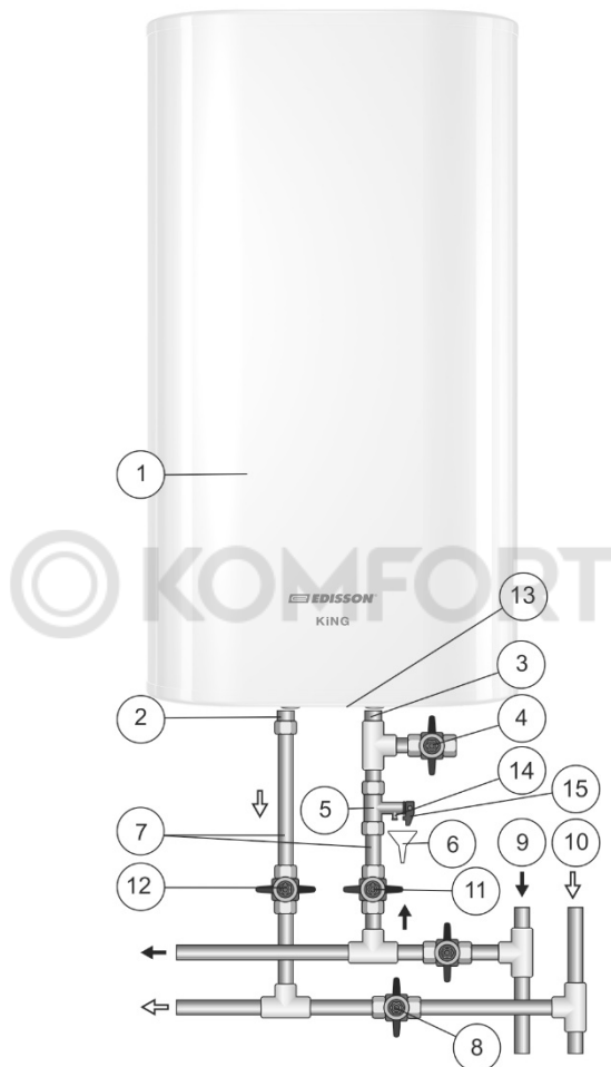
Рисунок 1. Схема подключения ЭВН к водопроводу сверху и снизу
