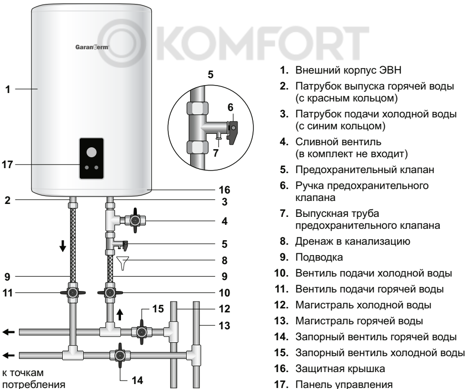
Рисунок 2. Схема подключения ЭВН к водопроводу.
