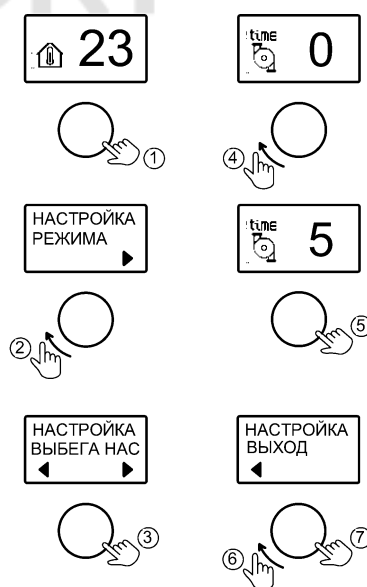
Рисунок 12. Настройка времени выбега насоса
