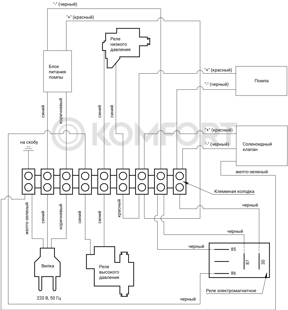
Рис. 14 Электрическая схема.
