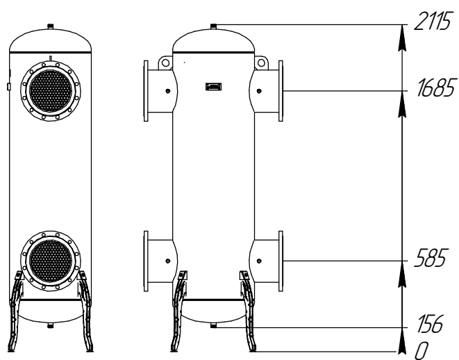
Монтажные размеры
