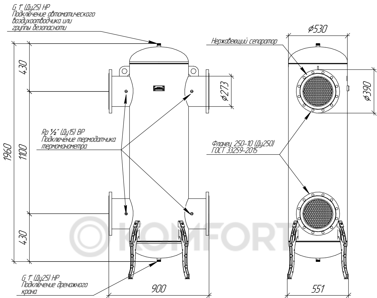
Монтажные размеры
