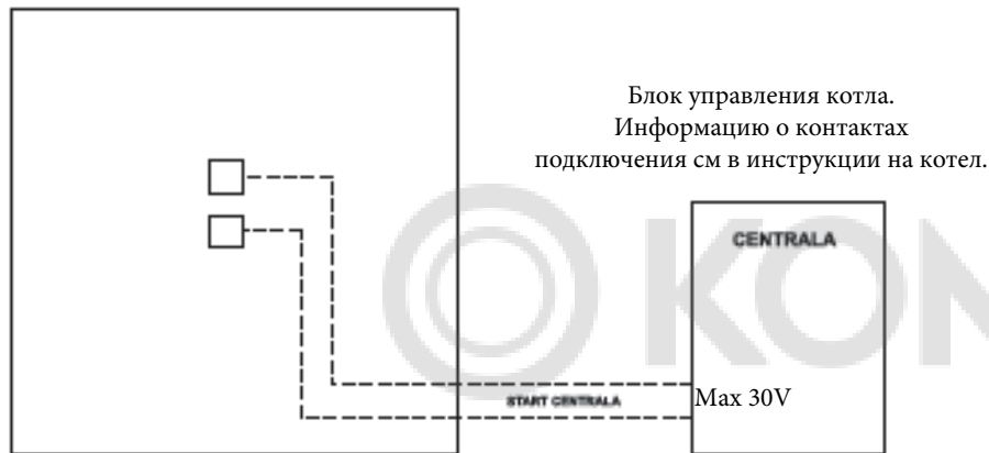
Электрическая схема соединения
