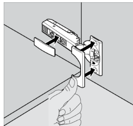
Установка заглушек
