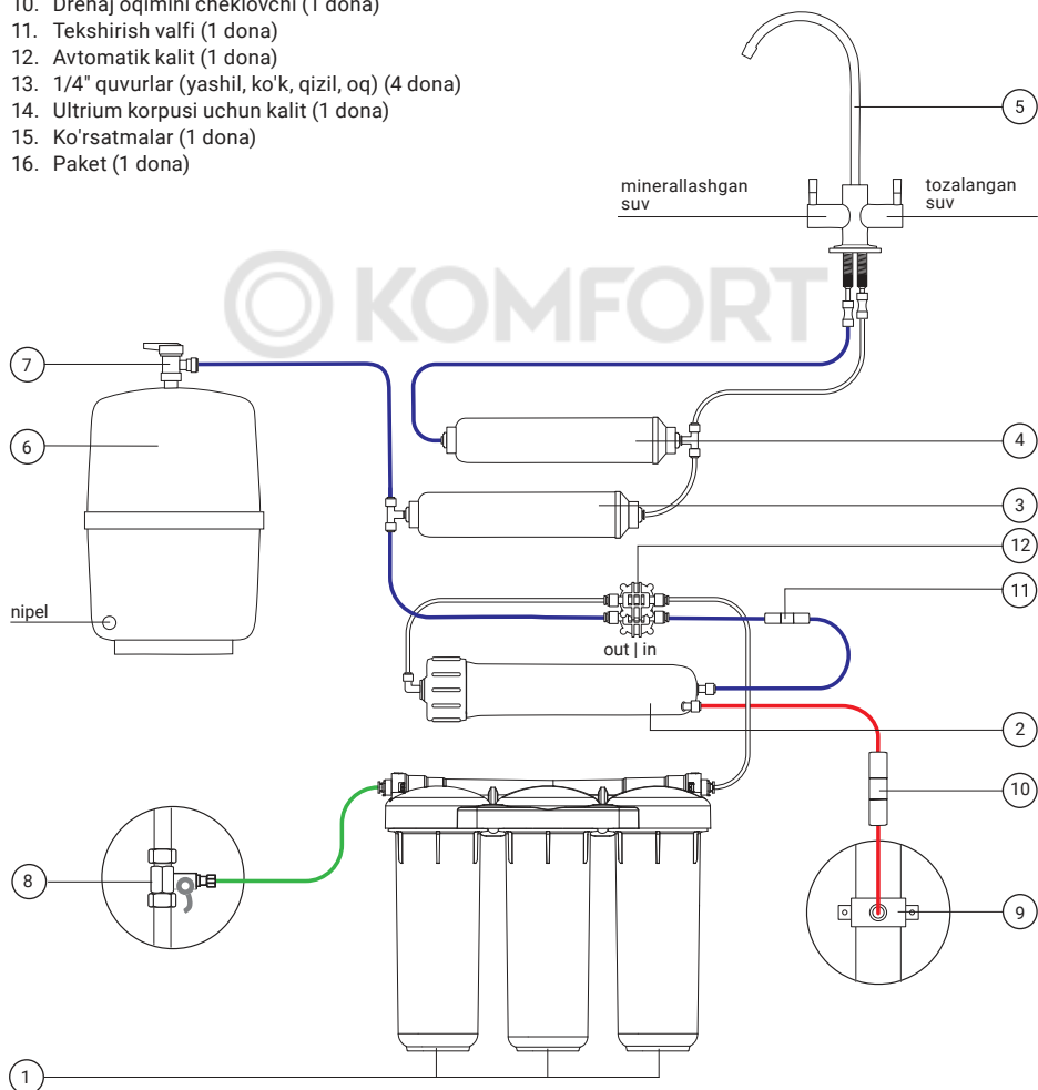
3 rasm Allegro M/Prestige M Geyserining avtomatik suv o'tkazgichi bilan ulanish sxemasi.
