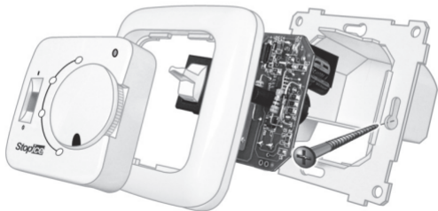
Рис. 3. Сборка терморегулятора
