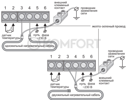
Рис. 4. Схема подключения терморегулятора TP 140 к трехпроводной электрической сети
