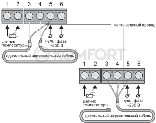
Рис. 5. Схема подключения терморегулятора TP 140 к двухпроводной электрической сети
