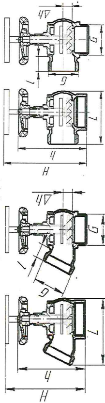
Исполнение 1: КПЛМ, КПЧМ, КПКМ, КПКМ Исполнение 2: КПЛМ, КПЧМ, КПКМ, КПКМ Рисунок 1—Внешний вид клапанов угловых моделей КПЛ, КПЧ, КПК и КПЛМ, КПЧМ, КПКМ
