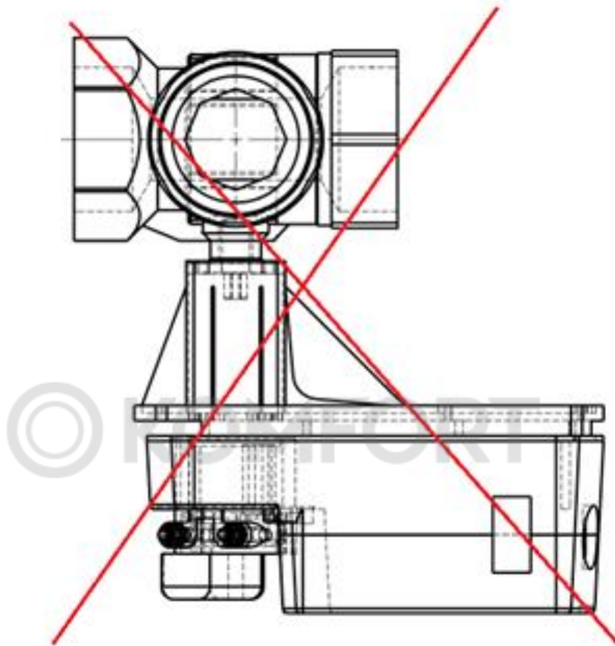
Рисунок А.1 – Недопустимое монтажное положение крана с электроприводом
