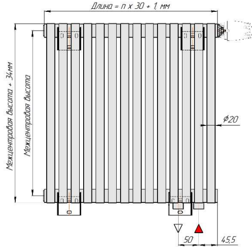
Присоединительная резьба - G 1/2" внутр.
