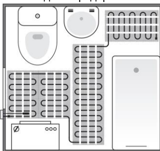
Рисунок 2 – Пример укладки нагревательного мата.
