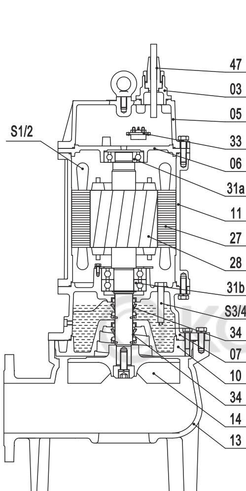
VSV 5,5–7,5 кВт
