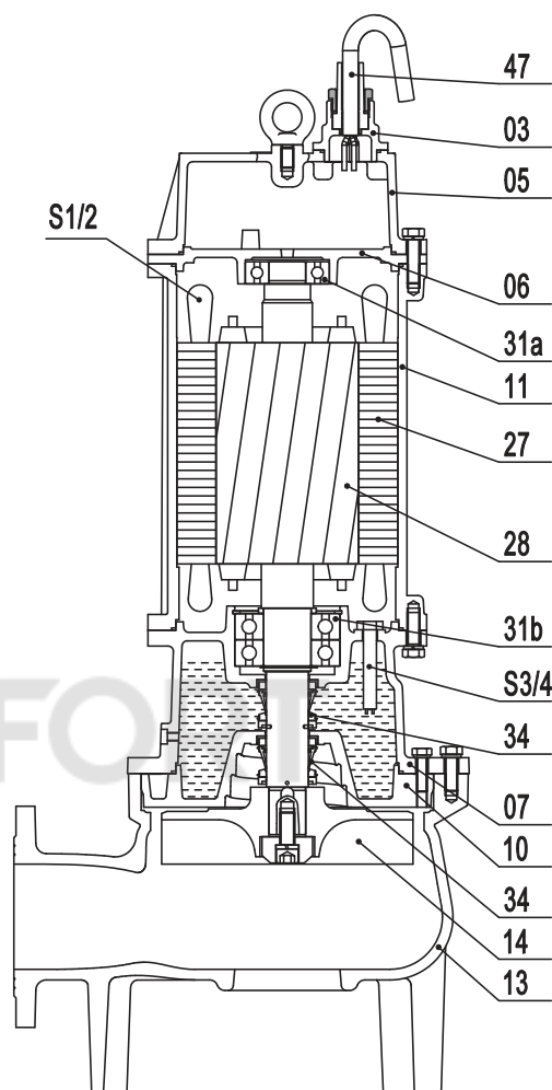
VSV 11,0 кВт
