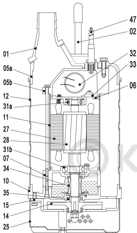
APV.09 1,5-2,2 кВт
