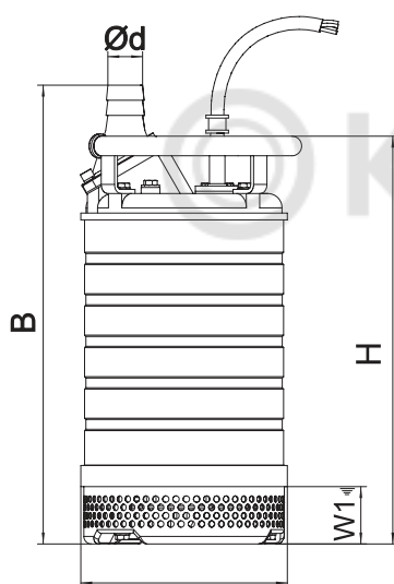
ØD 3,7–5,5 кВт
