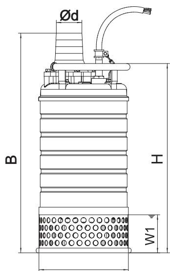
ØD 7,5–15 кВт
