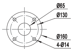
Размеры напорного патрубка насоса
