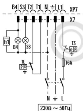
Электрическая схема горелки
