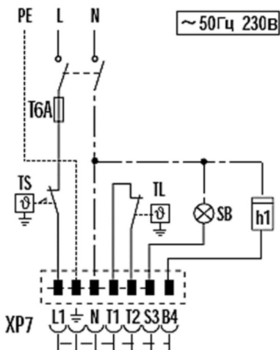
Электрическая схема горелки
