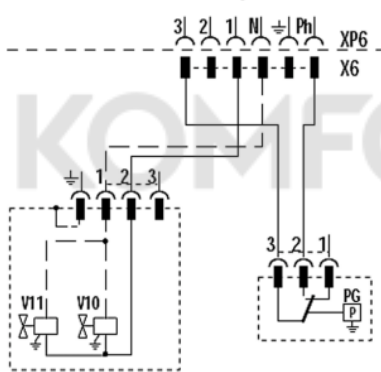
Электрическая схема газового мультиблока
