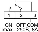
Рисунок 4 — Схема подключения нагрузки
