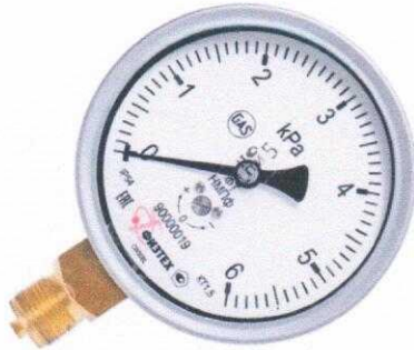
Рисунок 5 – Приборы коррозионностойкие
