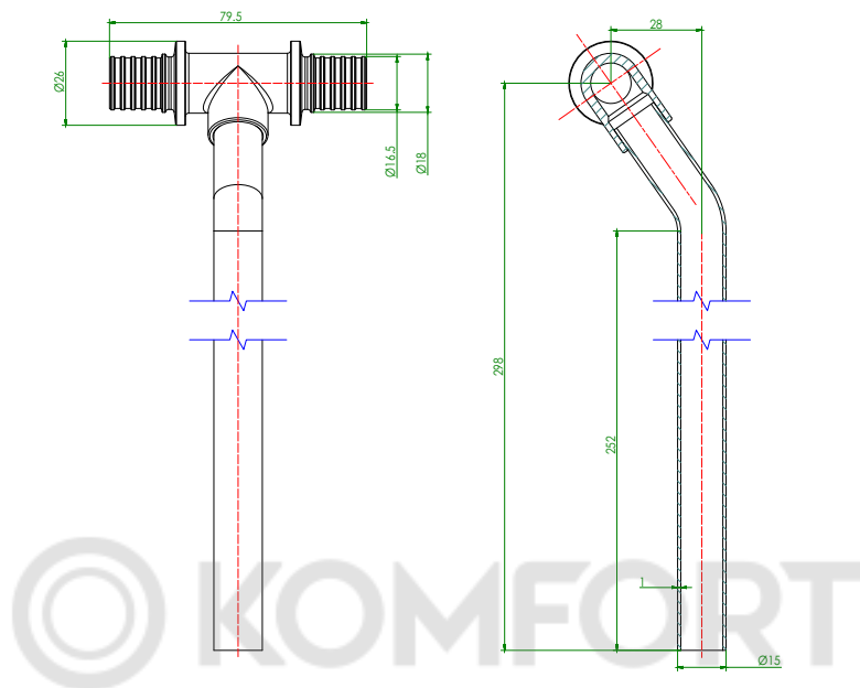
Рисунок 1. Основные габариты аксиальных фитингов ARROWHEAD
