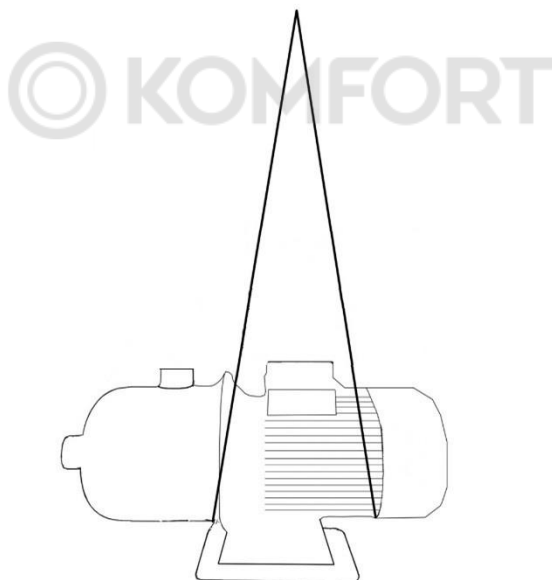
Рис. 2 Правильный подъем оборудования
