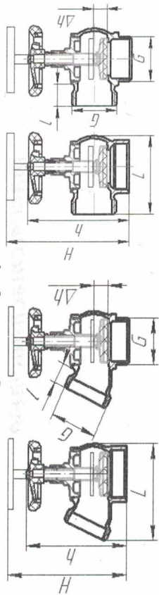
Исполнение 1: КПКМ, КПК, КПКМ Исполнение 2: КПКМ, КПКМ, КПКМ Рисунок 1 – Внешний вид клапанов угловых моделей КПКМ, КПК, КПК и КПКМ, КПКМ, КПКМ
