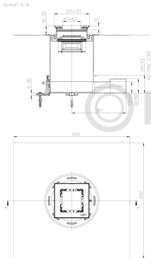
Рис. 2. Трап HL541I.
