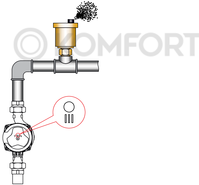
Рис.2 Удаление воздуха из корпуса насоса.
