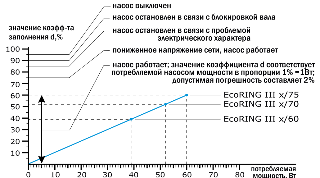
Рис.15 Зависимость коэффициента заполнения от состояния насоса.
