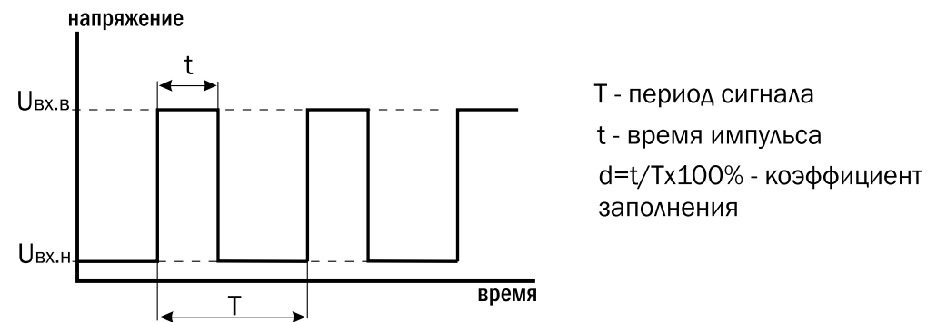
Рис.13 Характеристики ШИМ-сигнала.
