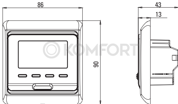
Рис. 2 Габаритные размеры терморегулятора
