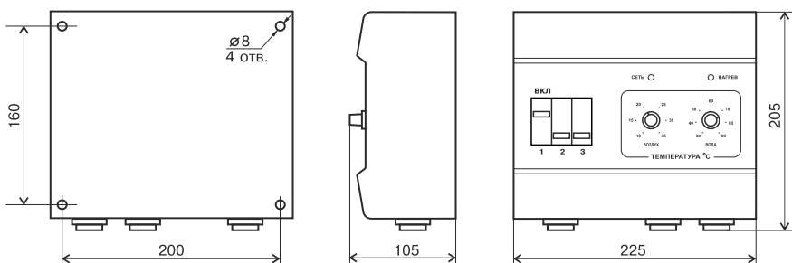
Рис.1 Габаритные и установочные размеры панели управления
