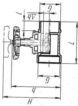
Рисунок 2 – Внешний вид прямоточной модели КПКЛ, КПКП и КПКЛ.
