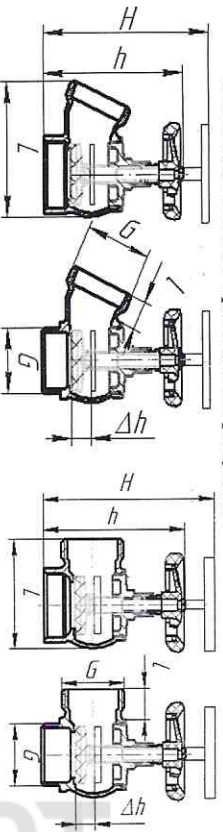
Рисунок 1 – Внешний вид клапанов угловых моделей КТЧМ, КТЧК, КТЧП и КТЧМ, КТЧМ, КТЧК, КТЧМ
