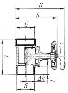
Рисунок 1 – Внешний вид клапанов угловых моделей КТЧМ, КТЧК, КТЧП и КТЧМ, КТЧМ, КТЧК, КТЧМ
