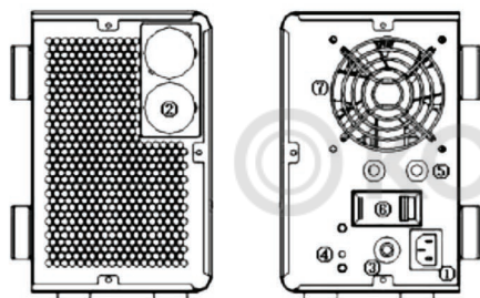
Серия PSW-HW
