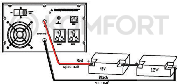
Схема подключения аккумуляторных батарей U=24V . Модель PSW-H 1600 Вт
