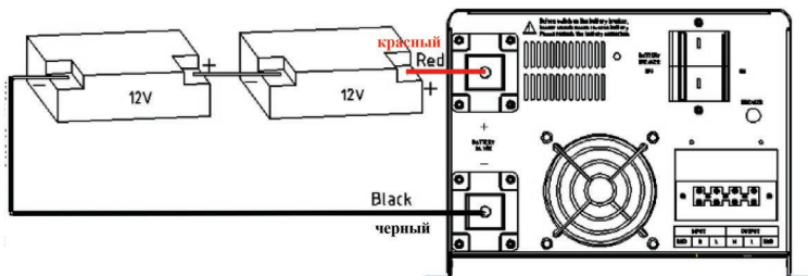
Схема подключения аккумуляторных батарей U=24V . Модель PSW-HW 2500-3500 Вт
