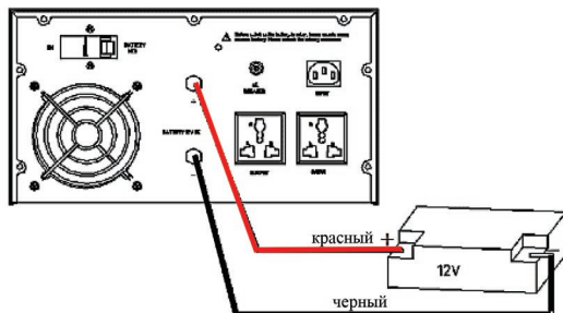
Схема подключения аккумуляторных батарей U=12V . Модель PSW-H 300-1000 Вт
