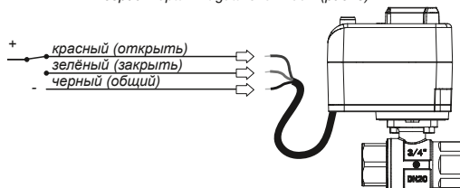
Электрическая схема подключения крана с электроприводом серии Neptun Bugatti Click 12B и Click 18B (рис. 4)
