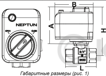
Габаритные размеры (рис. 1)
