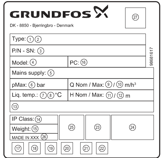
Նկար 2 Ֆիրմային վահանակ
