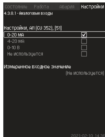
Рис. 81 Аналоговые входы
