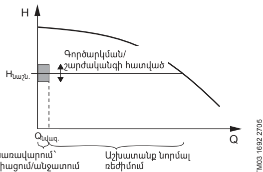
Նկար 70 Գործարկման/շարժական գիծ
