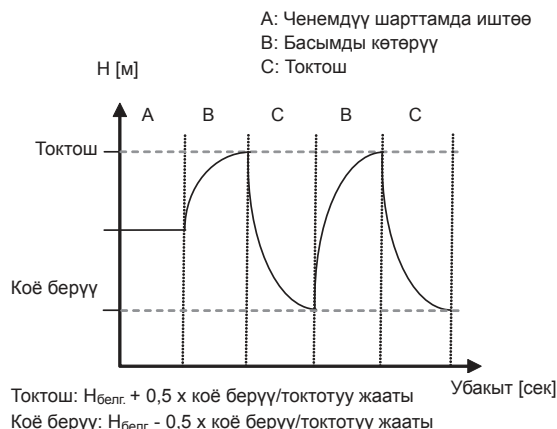
71-сур. Күйгүзүү/өчүрүү шарттамында иштөө
