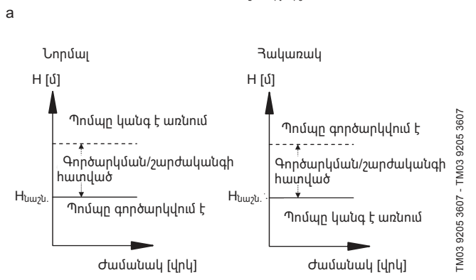
Նկար 55 Նորմալ և հակառակ կառավարում
