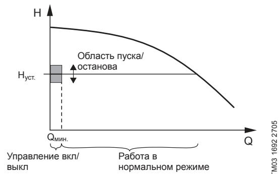
Рис. 70 Область пуска/останова
