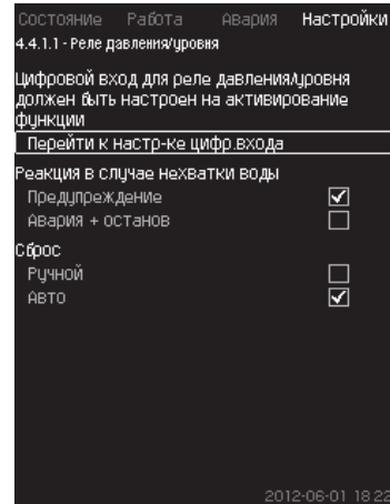
Նկար 105 Ճնշման/մակարդակի ռելե
