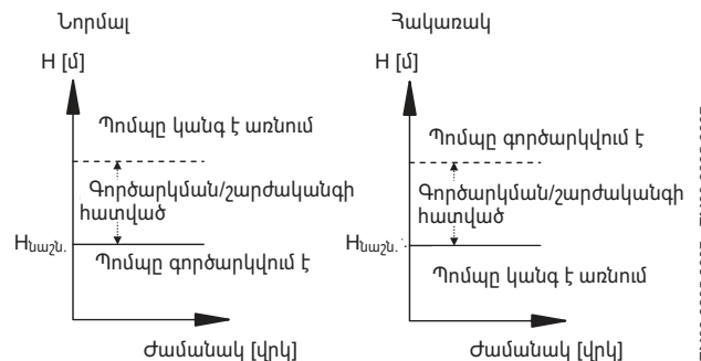
Նկար 55 Նորմալ և հակառակ կառավարում
