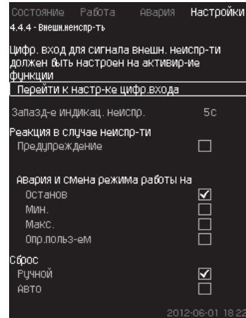
Նկար 110 Արտաքին անսարքություն
