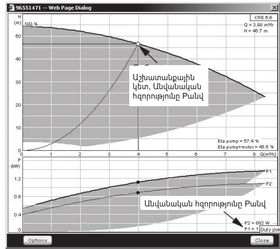
նկար 96 Անվանական հզորության ցուցումը P անվանական Q անվանական և H անվանական - պոմպերի անվանական աշխատանքային կետ և, որպես օրինակ, դա ամենաբարձր ՕԳԳ-ով կետն է:
