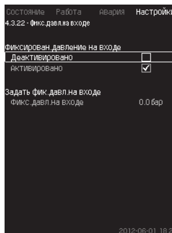
Рис. 98 Фикс.давл.на входе
