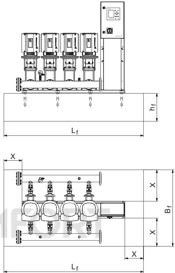
Рис. 7 Հիմնատակ
