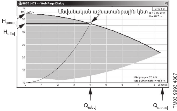
նկար 93 Ցուցումը Q անվանական , H անվանական , H առավելագույն և Q առավելագույն
