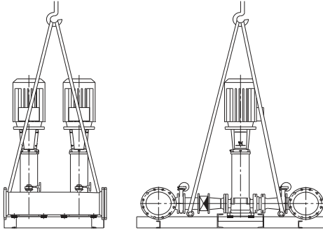
Նկար 4 Hydro MPC ձիշտ բարձրացում
