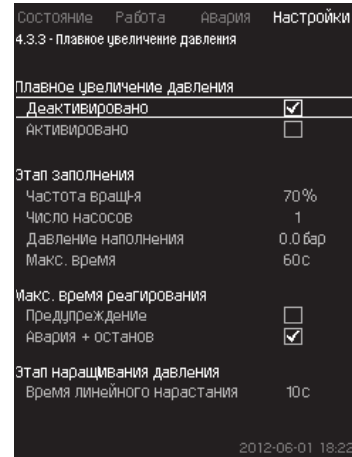
Նկար 75 Ճնշման աստիճանաբար ավելացում
