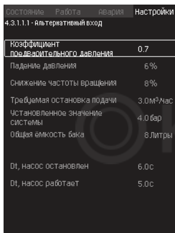
Նկար 74 Այլընտրանքային մուտք
