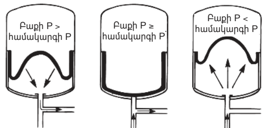
Նկար 5 Թաղանթային ձնշումային բաք (P՝ ձնշում)
