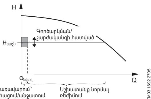
Նկար 70 Գործարկման/շարժական գիծի հատված
