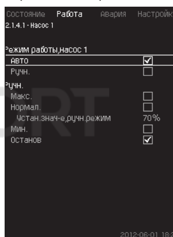
Рис. 34 Насос 1 - 6
