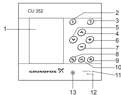
Рис. 9 Панель управления
