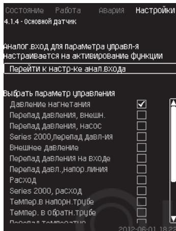
Рис. 48 Основной датчик
