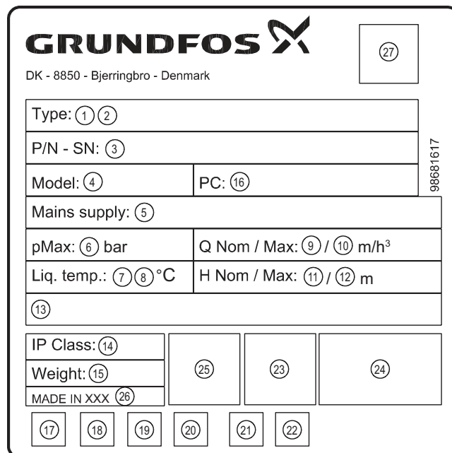
Рис. 2 Фирменная табличка
