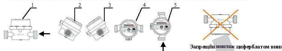
Рисунок 2. Возможные варианты установки счётчика при монтаже
